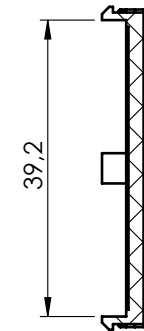
SECTION A-A
