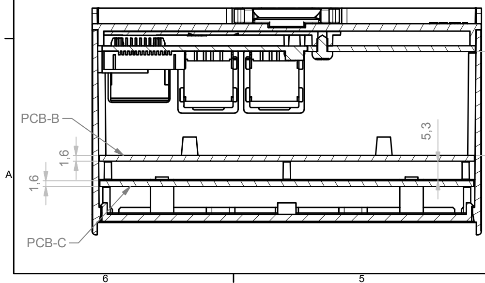
A-A (1:1)
