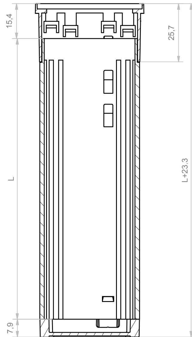
A-A (1:1)
