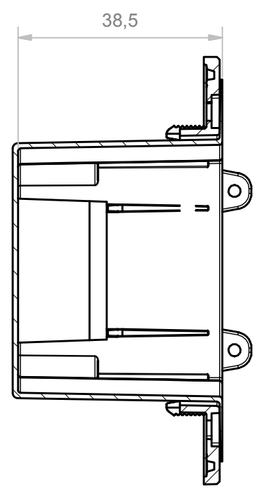
A-A (1 : 1)
