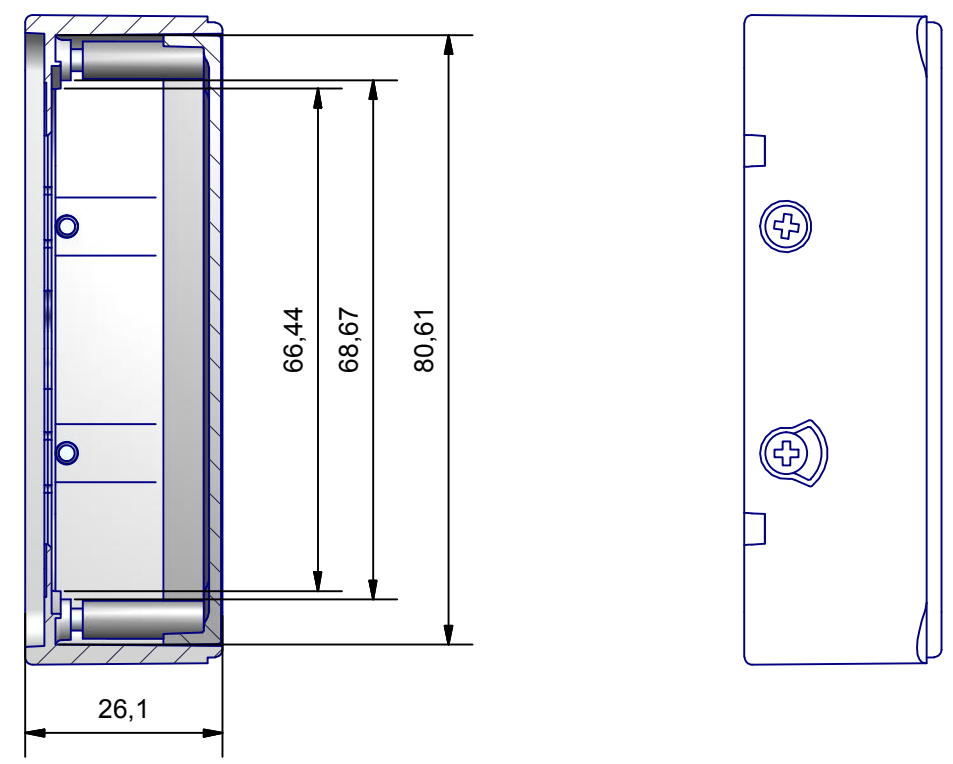
A-A (1:1)
